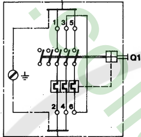
WIRING DIAGRAM FOR SCHALTPLAN FÜR 80800 KA AND/UND KT
