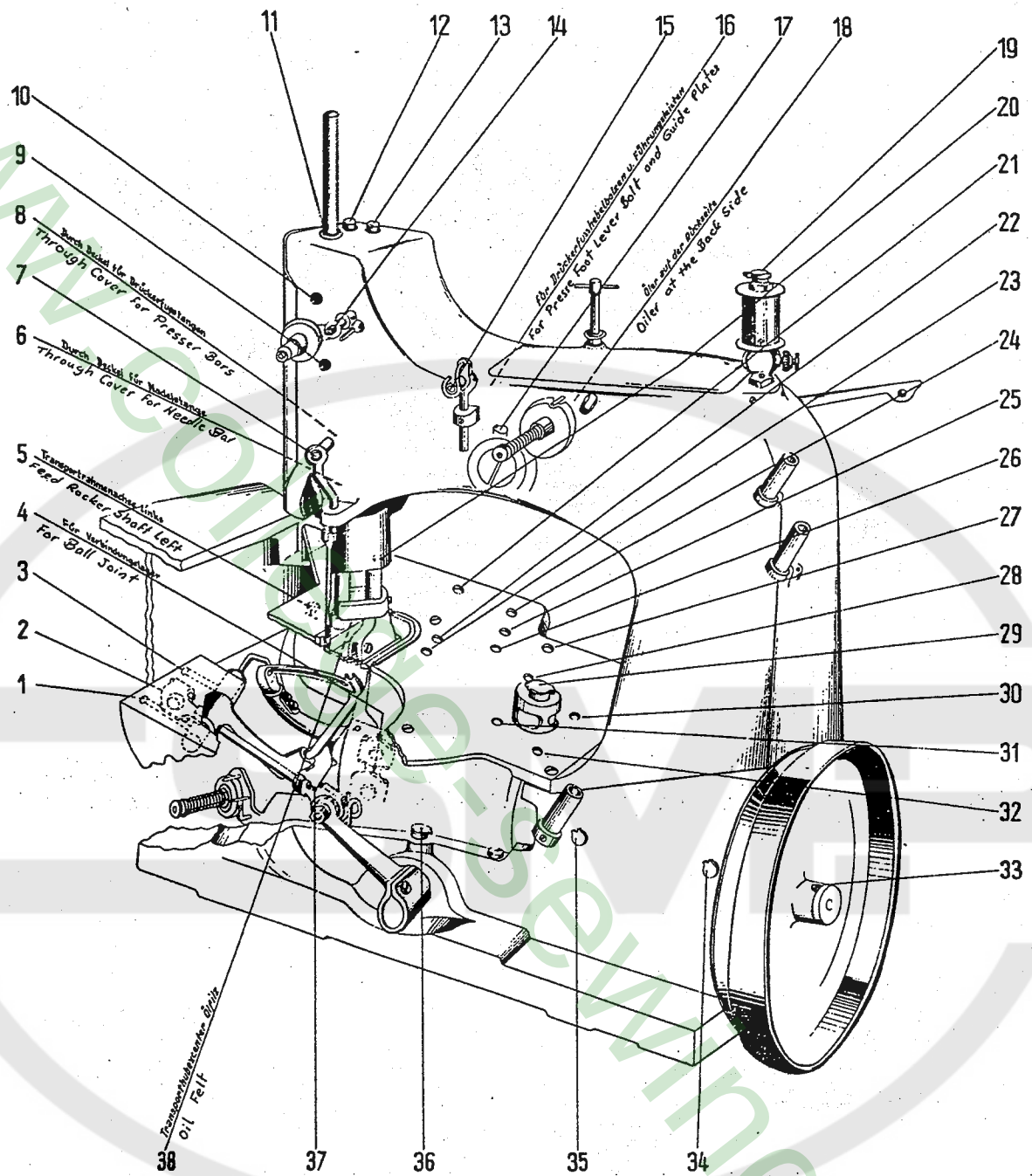
ÖL-DIAGRAMM
