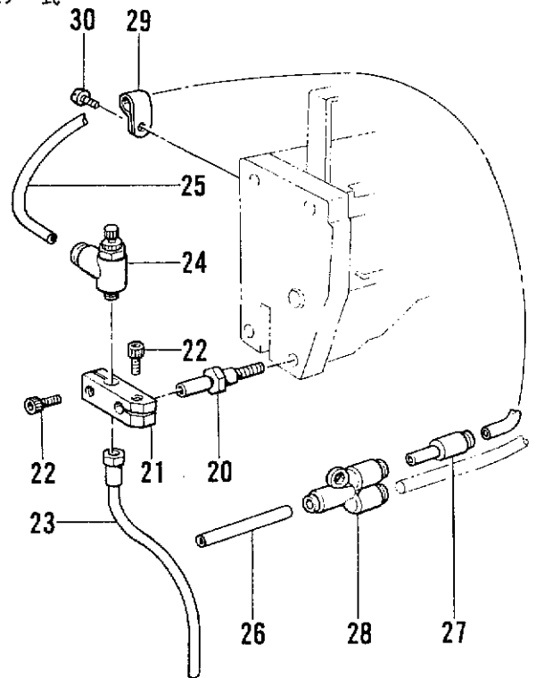
エア式
